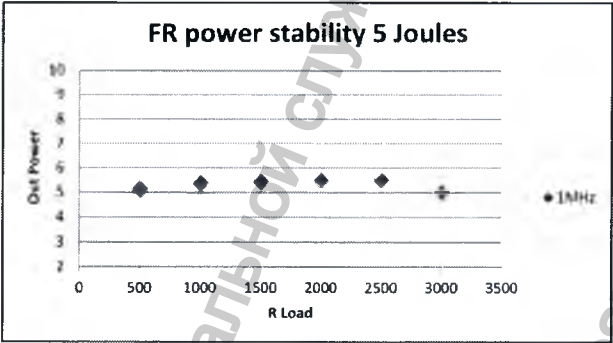
Рис. 6.15: Стабильность мощности V-FR
