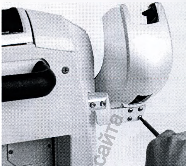
Рис. 5.4. Монтаж люльки
